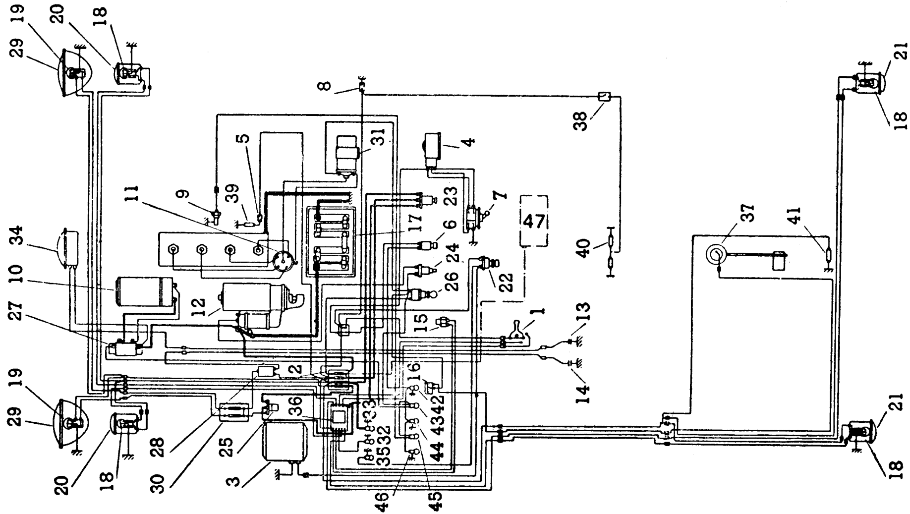
SCHEMA IMPIANTO ELETTRICO
